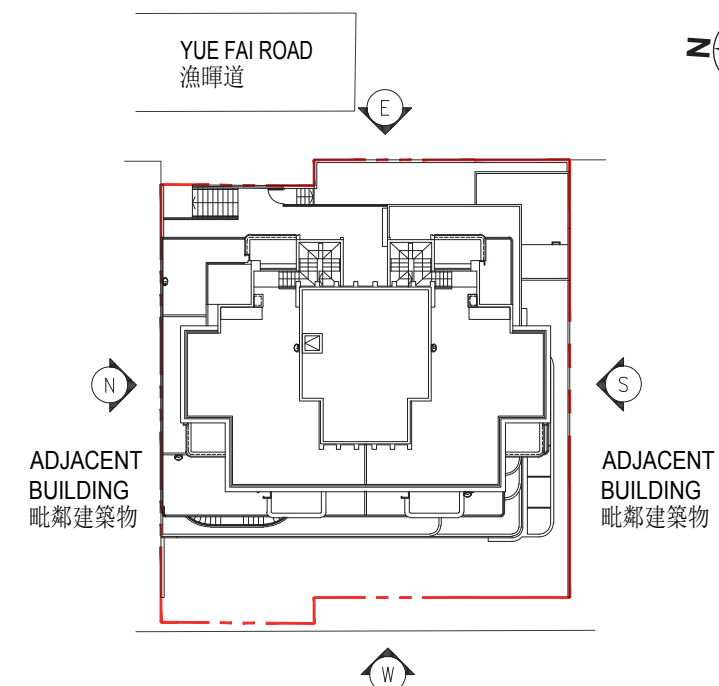
索引圖 Key Plan
